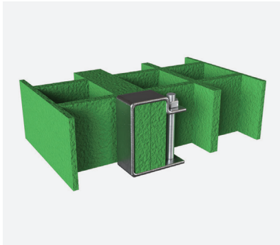
C Clip
