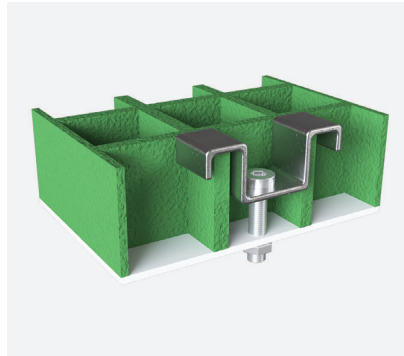
M Clip
